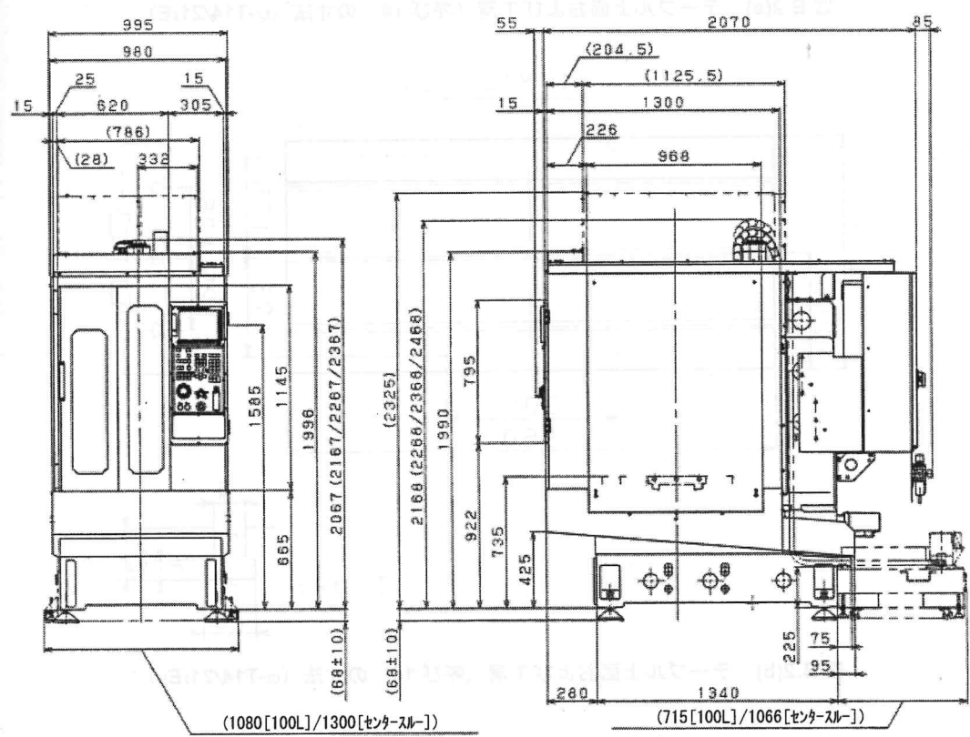
図 B.1(c) 機械外観および寸法 ( \alpha -T14/21iEs)
