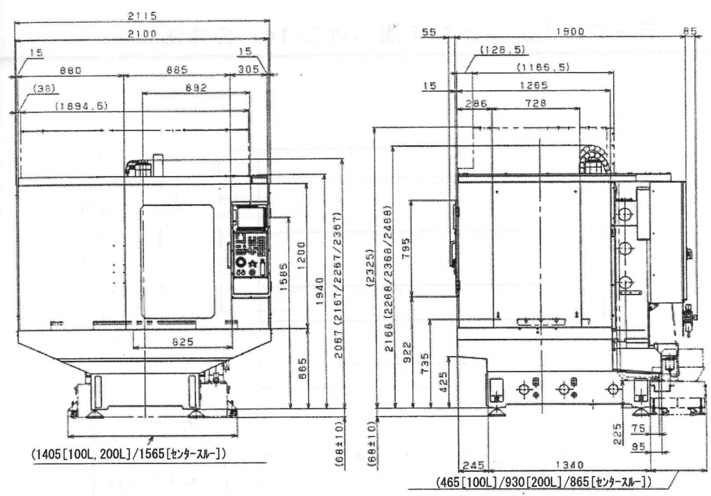
図 B.1(b) 機械外観および寸法 ( \alpha -T14/21iEL)
